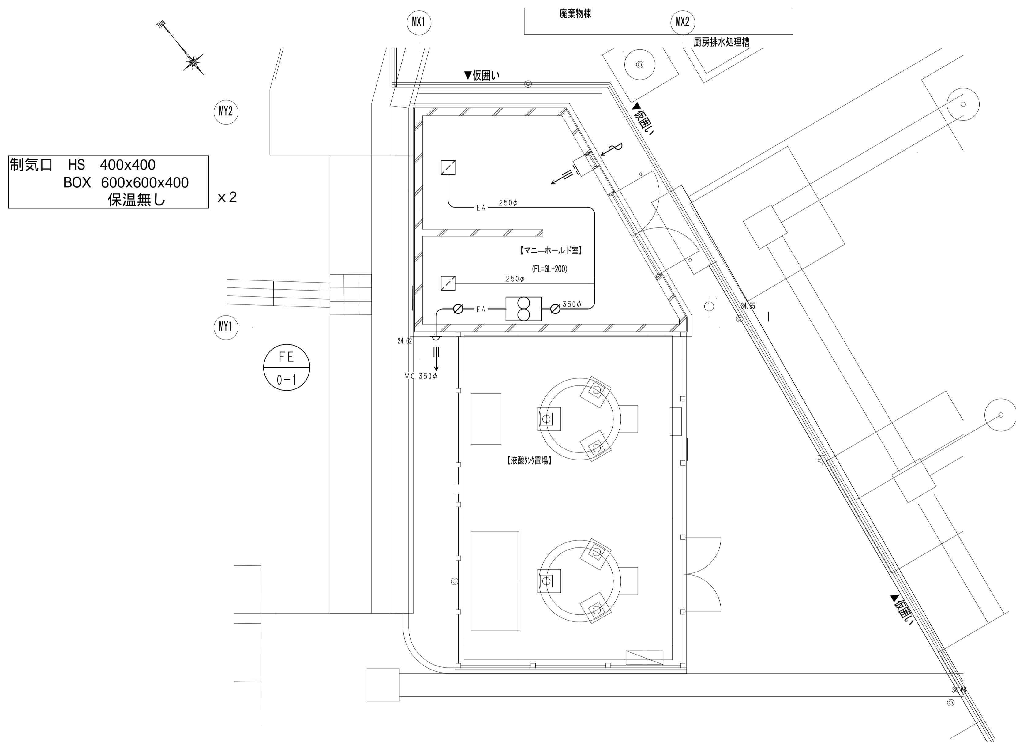
マニホールド室 ダクト詳細図
